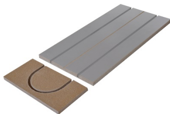
Rohrabstand 250 mm
