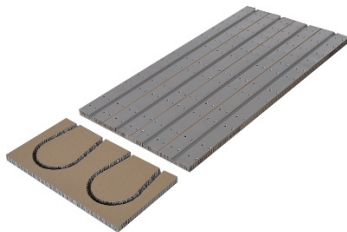
Rohrabstand 250 mm
