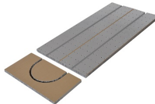
Rohrabstand 125 mm
