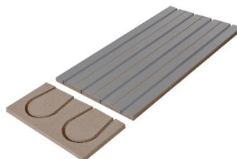
Rohrabstand 125 mm
