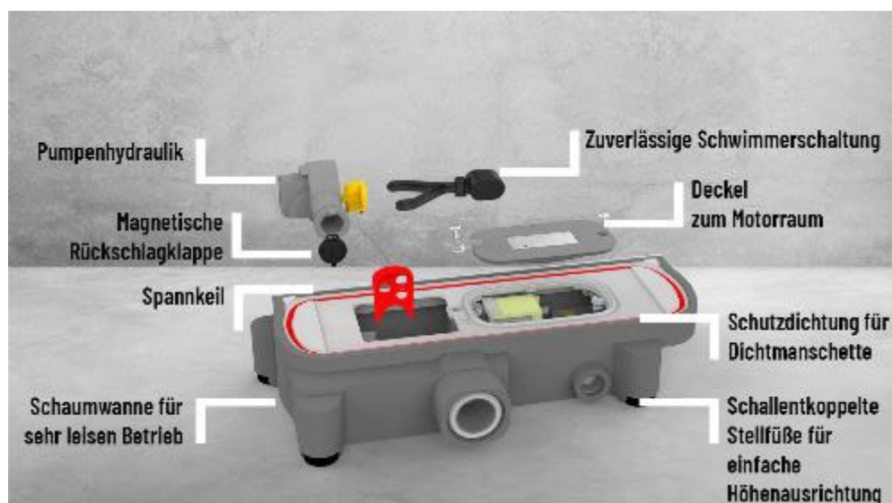
Abb. 3: Der Plancofix Connect: Eine kleine Pumpe im Bodenablauf fördert das verbrauchte Duschwasser leise und zuverlässig in das vorhandene Abwassersystem und ermöglicht so eine barrierefreie Dusche im Bestand. (Bild: Jung Pumpen GmbH)
