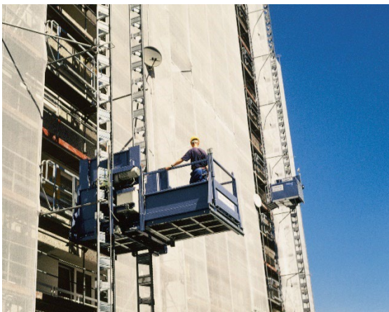
GEDA 1500 ZP
